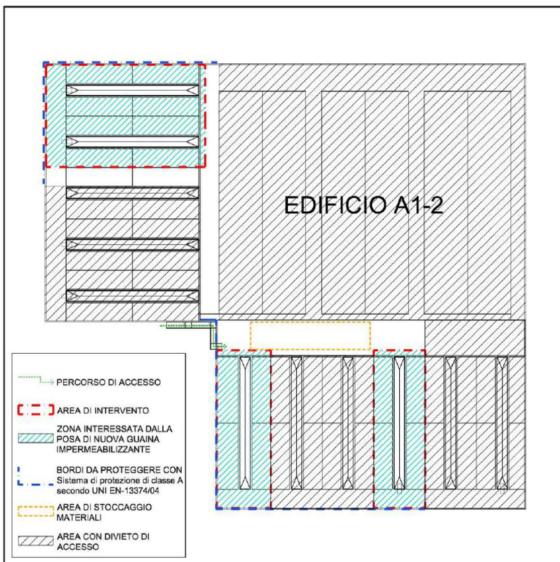
SCHEMA AREA DI CANTIERE
